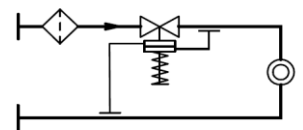
Установка регулятора на подающем трубопроводе
